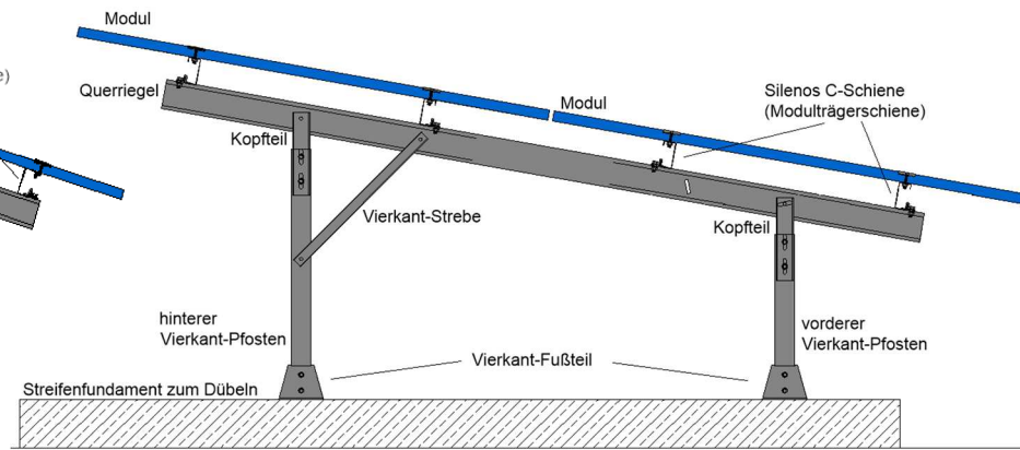
2-Pfosten-System zum Aufdübeln auf Streifenfundamente
