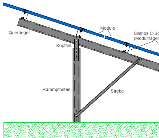
1-Pfosten-Rammsystem
