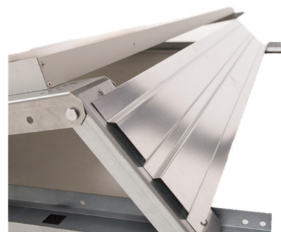
Rückblech bei Süd-Aufständerungen
