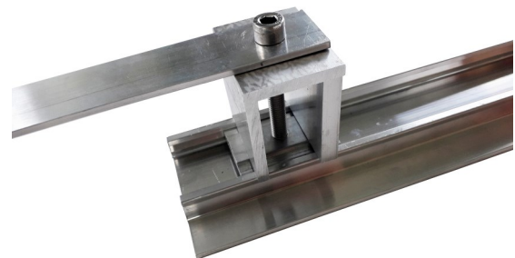
Abrutschsicherung über den First
