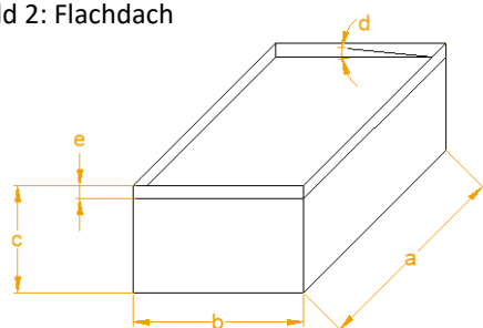
Bild 2: Flachdach
