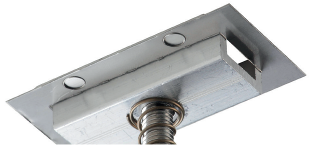
optional: Mittelklemmen-Set mit Erdungsplättchen
