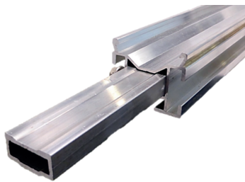
ZELOS Profil mit innenliegendem ZELOS Schienenverbinder
