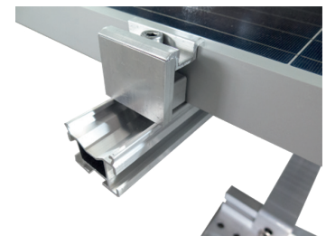
Mittelklemmen-Set + Ausgleichsprofil zum Einklicken
