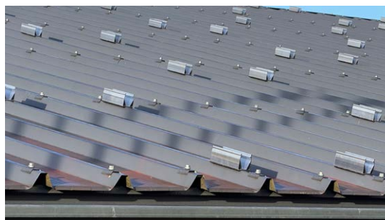
CHRONOS Trapez beta mit Modulabstand zur Hochsicke von 45 mm
